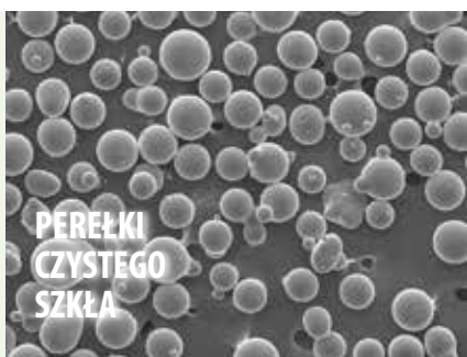
Obraz perełek szkła pod mikroskopem skaningowym
