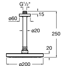
Vintage Ramię sufitowe z deszczownicą o średnicy 200 mm NR REF. A5B9550C00
