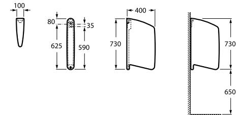
SERIA Wing, przegroda pisuarowa NR REF. A387090000
