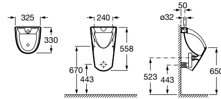
SERIA Chic NR REF. A35945N000 ZASILANIE z góry
