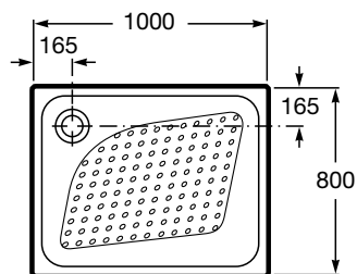
Frontalis brodzik ceramiczny NR REF. A373581..0
