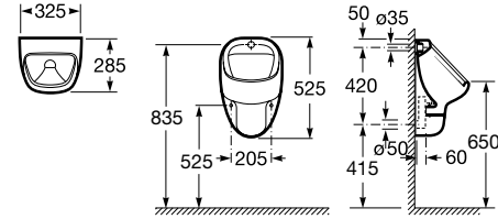
SERIA Urinett bez pokrywy NR REF. A359093..5 ZASILANIE z tyłu
