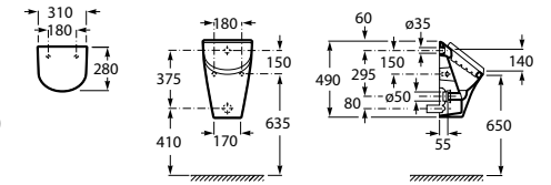
SERIA Nexo bez pokrywy NR REF. A35364L..0 ZASILANIE z tyłu SERIA Nexo z pokrywą NR REF. A35364K..0 ZASILANIE z tyłu
