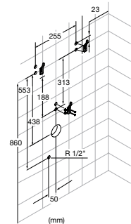
SERIA Urinett bez pokrywy NR REF. A359093..5 ZASILANIE z tyłu
