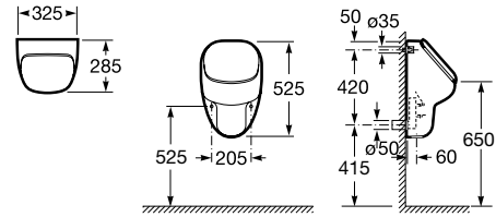
SERIA Urinett z pokrywą NR REF. A359097..0 ZASILANIE z tyłu
