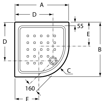
Easy Corner Brodzik ceramiczny NR REF. A374798..1 800x800 mm NR REF. A374797..1 900x900 mm
