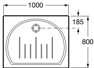
Happening brodzik ceramiczny NR REF. A373565000
