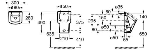
SERIA Hall NR REF. A35362E000 ZASILANIE z tyłu
