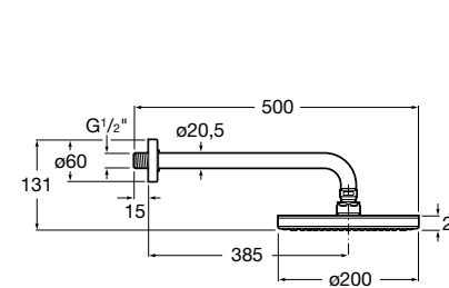
Vintage Recto Deszczownica o średnicy 200 mm z ramieniem NR REF. A5B9750C00
