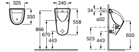
SERIA Chic NR REF. A35945O000 ZASILANIE z tyłu
