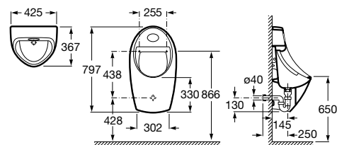
SERIA Euret 230 VAC NR REF. A35945M000 ZASILANIE z tyłu
