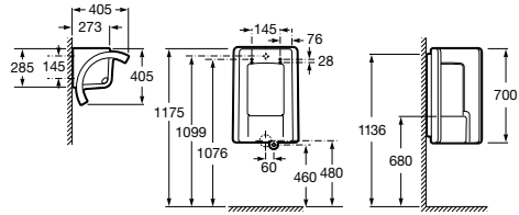
SERIA Site NR REF. A359601000 ZASILANIE z tyłu
