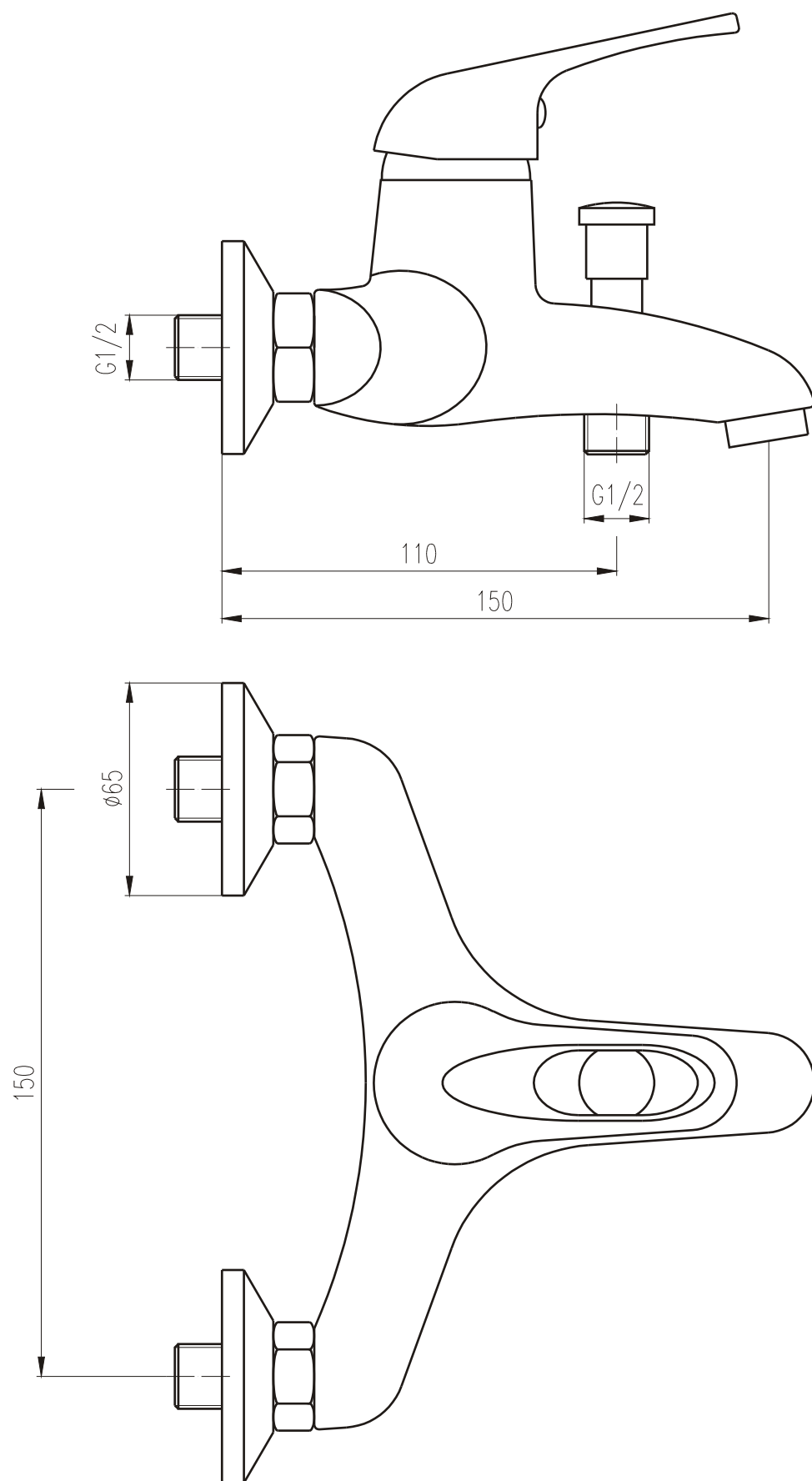
HAXE Jednouchwytowe tradycyjne Bateria wannowa ścienna KOD: BFH 011M
