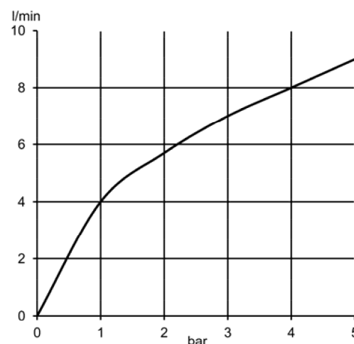
Diagram przepływu
