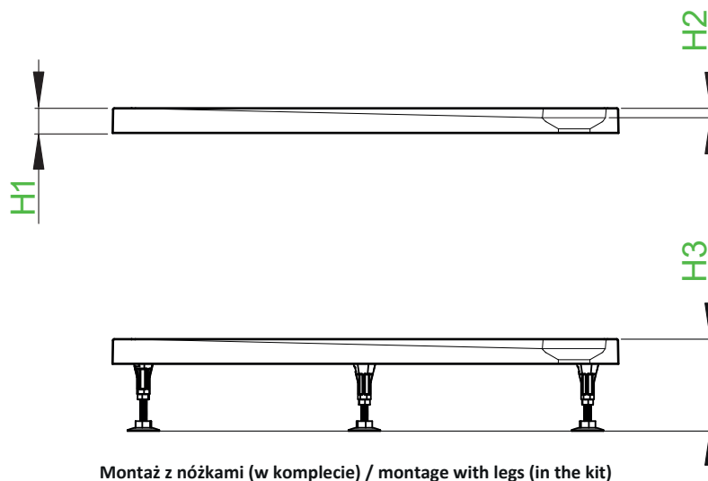
Montaż z nóżkami (w komplecie) / montage with legs (in the kit)
