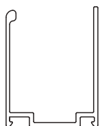
profil č. 7570
