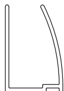
profil č. 7778
