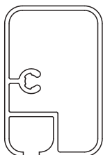
profil č. 7564
